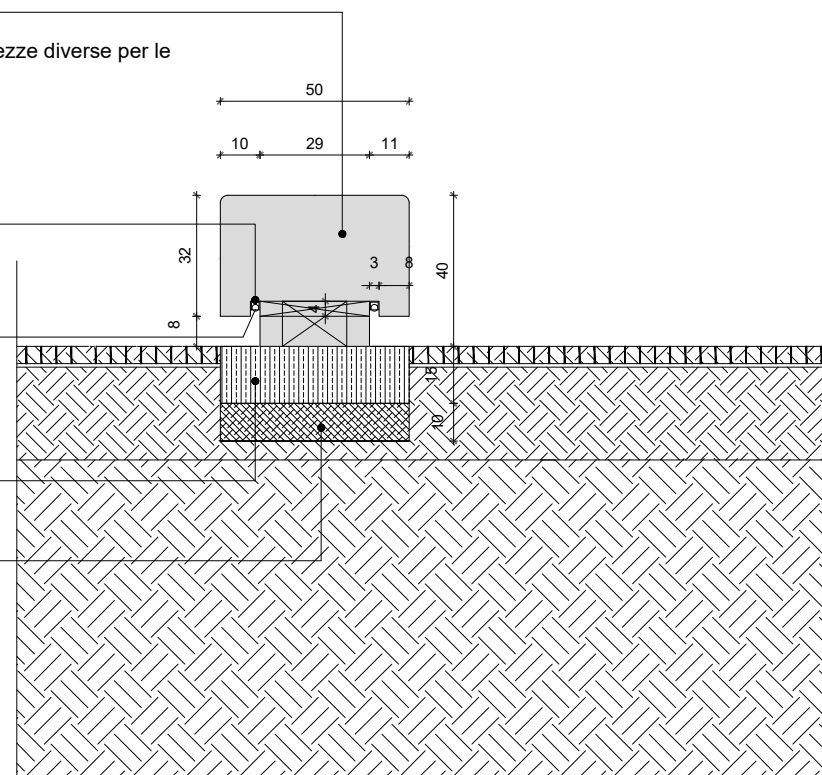
S02 DETTAGLIO S02 SEZIONE PANCA DECORATIVA SU PRATO ARMATO | Bam
