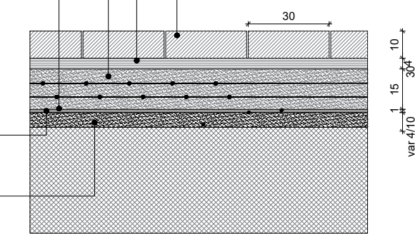
S07 DETTAGLIO S07 STRATIGRAFIA RAMPA CARRABILE Corso Como
