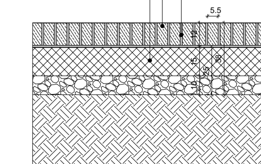
S05 DETTAGLIO S05 STRATIGRAFIA MATTONI A VISTA | Bam
