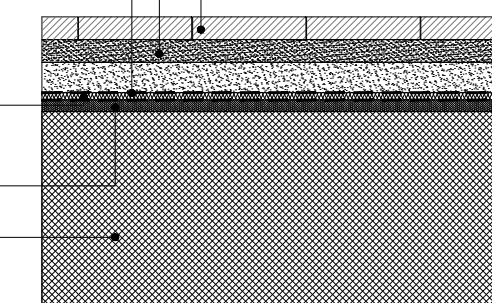
S09 DETTAGLIO S09 STRATIGRAFIA PAVIMENTAZIONE Piazza Alvar Aalto
