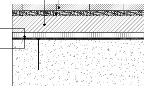
S08 DETTAGLIO S08 STRATIGRAFIA PAVIMENTAZIONE Piazza Gae Aulenti
