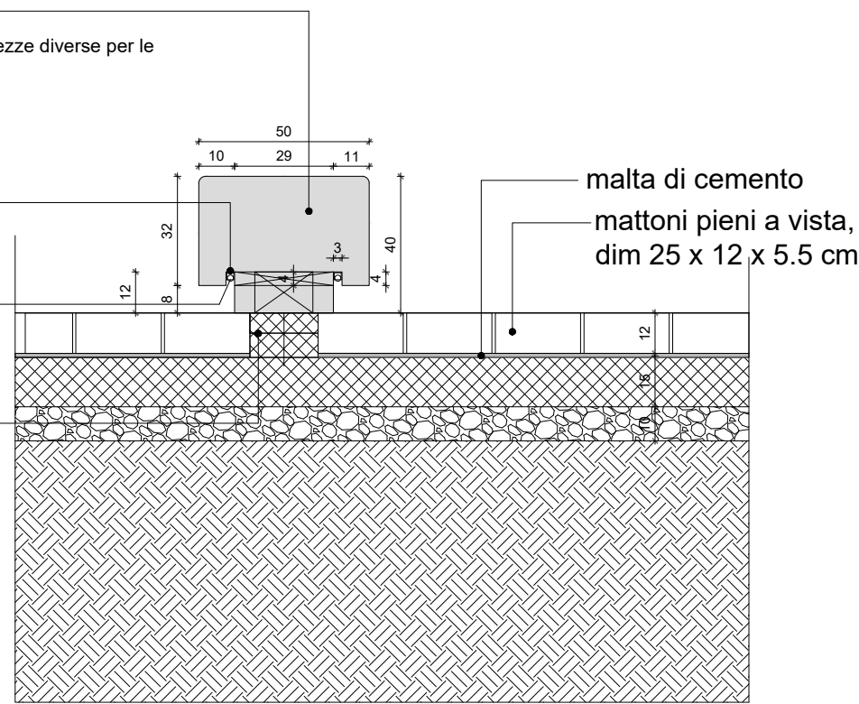
S01 DETTAGLIO S01 SEZIONE PANCA DECORATIVA SU MATTONI | Bam
