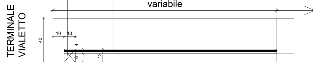
S03 DETTAGLIO S03 PROSPETTO PANCA DECORATIVA SU PRATO ARMATO | Bam
