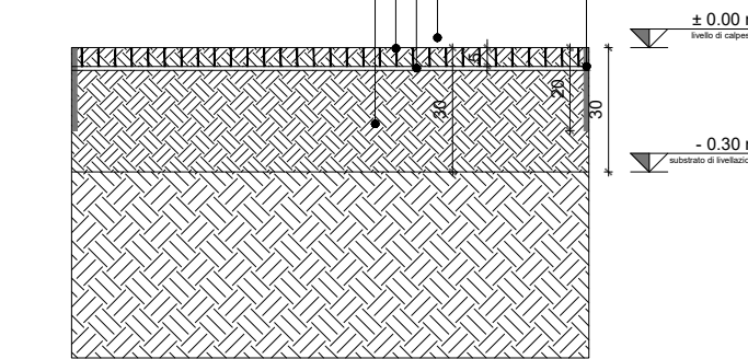
S04 DETTAGLIO S04 STRATIGRAFIA PRATO ARMATO | Bam
